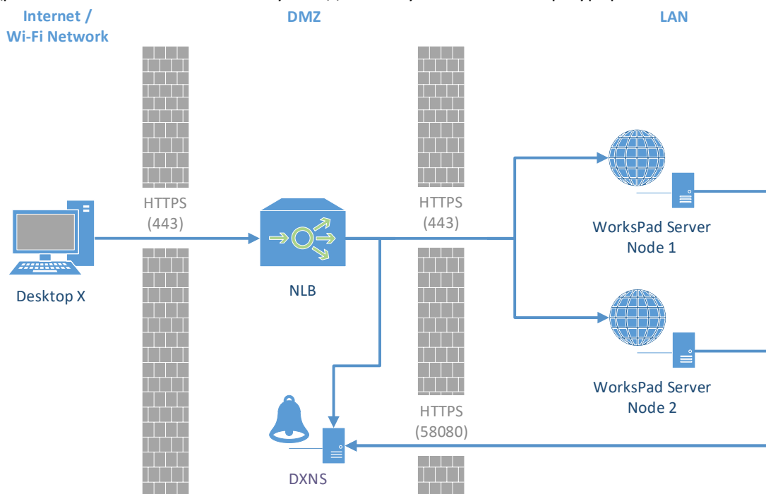
Пример размещения DXNS в DMZ
